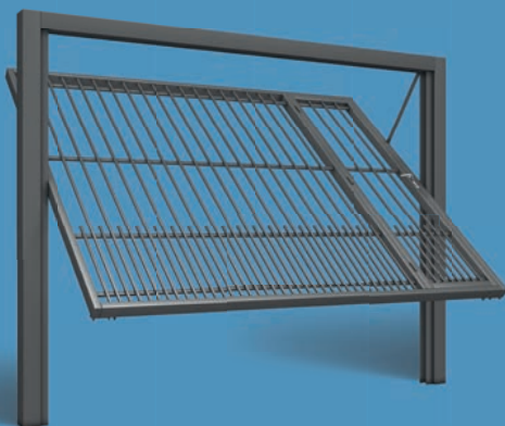
168. CONTRAPESO DE AÇO COM GRADE TUBULAR
