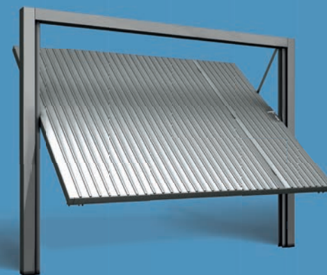
171. CONTRAPESO DE AÇO GALVANIZADO COM CHAPA FRISADA
