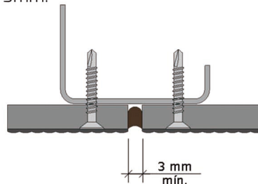
Junta de dilatação de no mínimo de 3mm de espessura.
