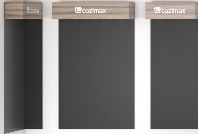
PAREDE 90 CANTO Ref. P-100067 L: 90 cm A: 230 cm P: 32,4 cm
