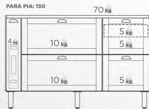
GABINETE L: 144,1 cm A: 91 cm P: 51,5 cm
