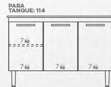
TANQUE L: 117 cm A: 91 cm P: 53,5 cm
