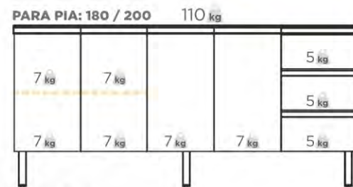
GABINETE L: 174 / 192 cm A: 84,8 cm P: 49,8 cm
