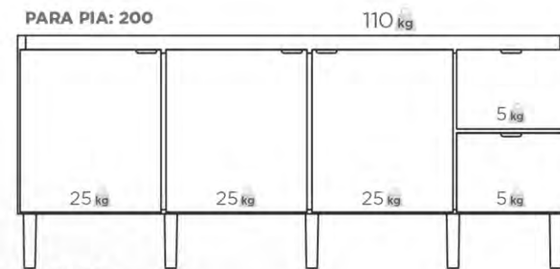
GABINETE L: 194 cm A: 78,7 cm P: 51 cm
