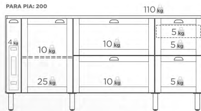
GABINETE L: 194,1 cm A: 91 cm P: 51,5 cm
