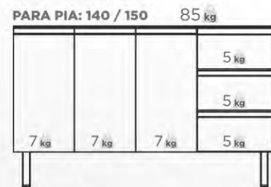
GABINETE L: 134,7 / 144,5 cm A: 84,8 cm P: 49,8 cm
