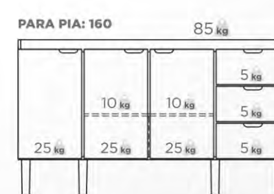
GABINETE L: 154 cm A: 85 cm P: 51,1 cm
