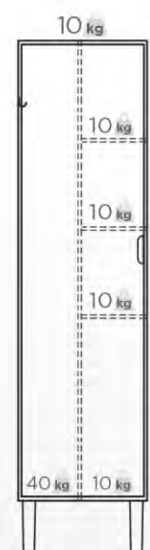
MULTIUSO L: 51 cm A: 192,4 cm P: 51,3 cm
