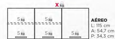
AÉREO L: 95,7 cm A: 54,7 cm P: 34,3 cm
