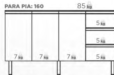
GABINETE L: 153,6 cm A: 84,8 cm P: 49,8 cm
