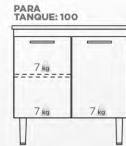
TANQUE L: 60,2 cm A: 92,9 cm P: 58,7 cm
