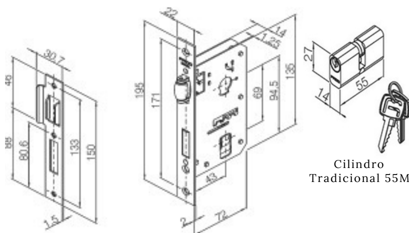
Máquina 45R e contra testa
