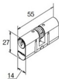
Cilindro ZM Concept 55MM Dimensões em milímetros
