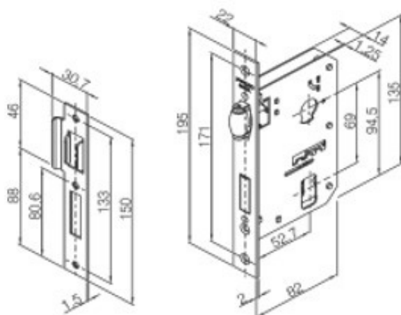
Máquina 55R e contra testa
